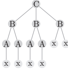
Fig. 20.3.2: 2(2 * 32 + 2 * 32 + \frac{2}{3} * 1) = 128\frac{2}{3}
