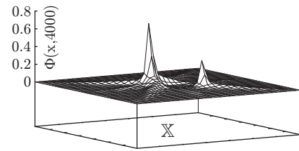
Fig. 1.18.10: \Phi(x, 4000)
