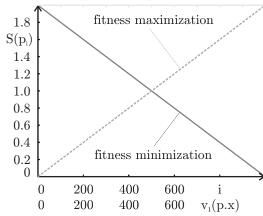
Fig. 2.9.1: v_1(p_i.x) = i
