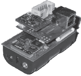
Fig. 29.7.1: BTNode
