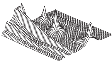
Fig. 20.1.7: t = 7
