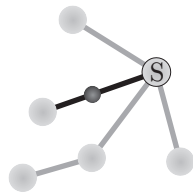
Fig. 29.11.1: Unicast
