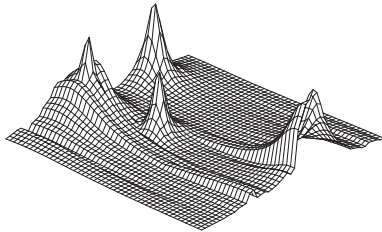
Fig. 20.1.5: t = 4
