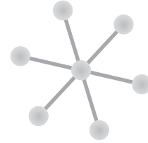
Fig. 29.3.3: star
