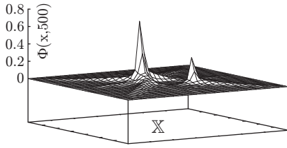
Fig. 1.18.7: \Phi(x, 500)
