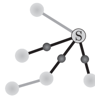
Fig. 29.11.2: Multicast
