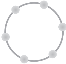
Fig. 29.3.4: ring
