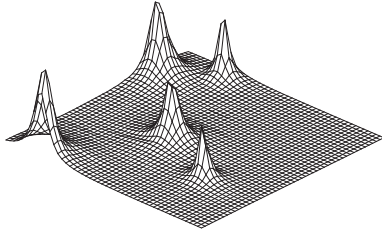
Fig. 20.1.1: t = 0
