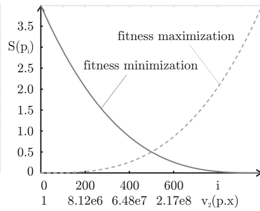
Fig. 2.9.2: v_1(p_i.x) = (i + 1)^3
