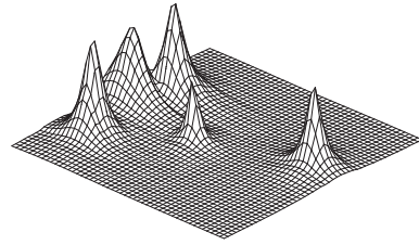
Fig. 20.1.2: t = 1
