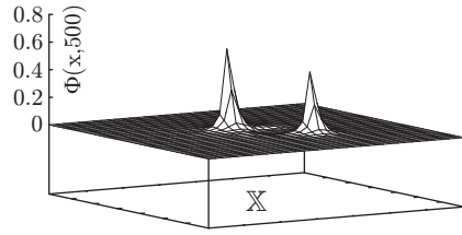
Fig. 1.17.7: \Phi(x, 500)
