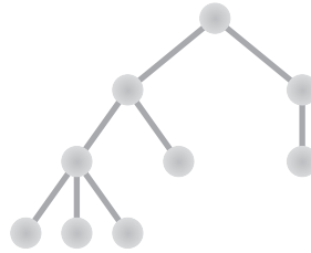
Fig. 29.3.5: hierarchy
