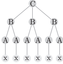
Fig. 20.3.1: 2(2 * 32 + 2 * 32 + 2 * 32) = 384
