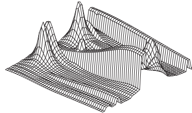
Fig. 20.1.4: t = 3
