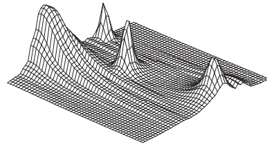
Fig. 20.1.6: t = 6
