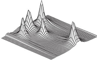
Fig. 20.1.3: t = 2
